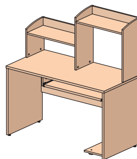
28S400 (изображено) 28S401 (зеркально) 1200x600x1354
