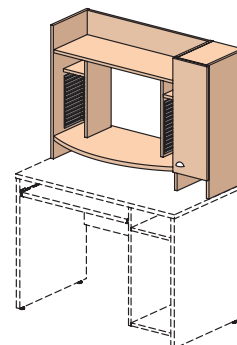
28P110 (изображено) 28P111 (зеркально) 994x400x714
